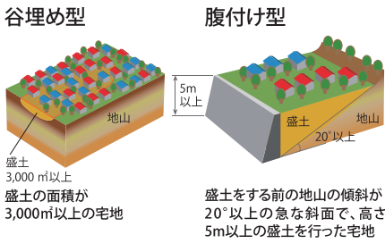
大規模盛土造成地(国土交通省「わが家の宅地安全マニュアル」より引用)
