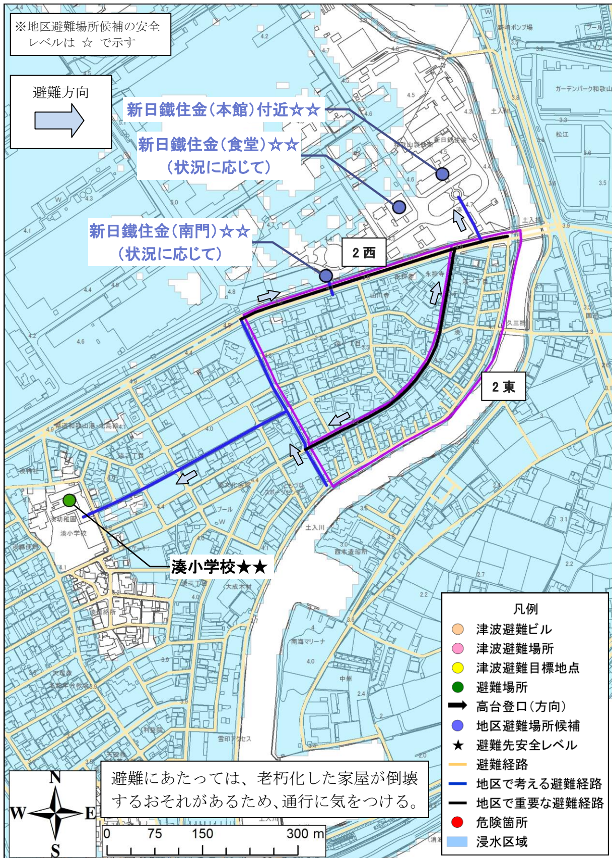
図 2 区東・西検討結果図
