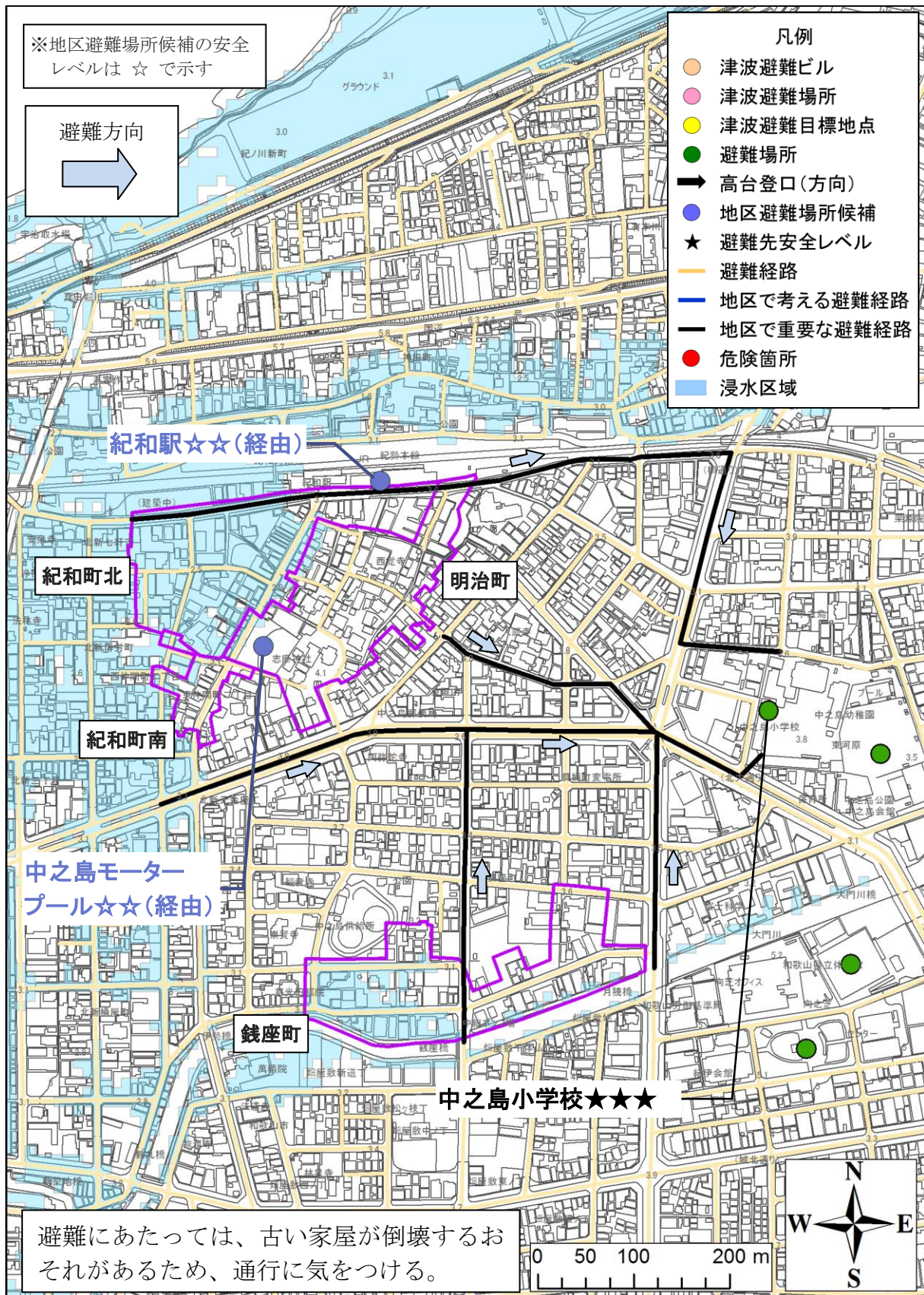
図 銭座町、紀和町北、紀和町南、明治町検討結果図
