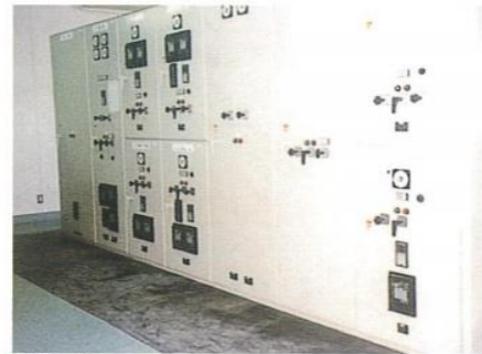
▲電気室
