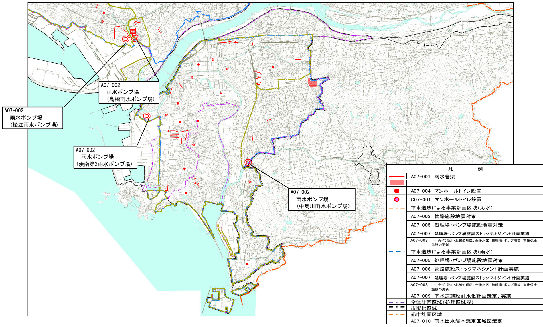
浸水対策、地震対策、改築更新事業対象箇所図(2/2)
