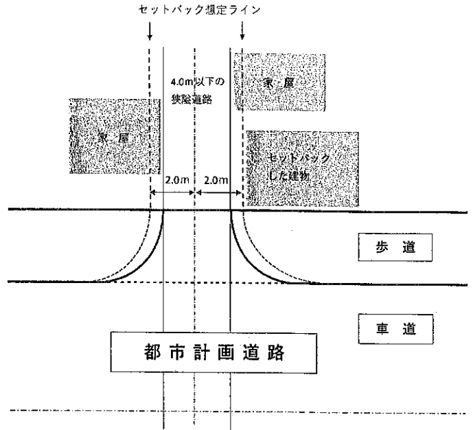
狭隘道路（市道）の先行拡幅を想定した取付部の整備
