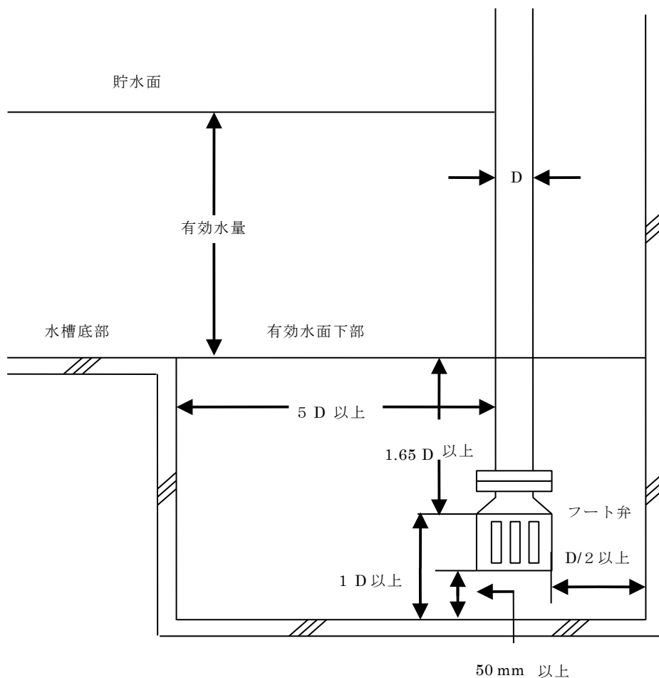
第13-5-1図 (地下又は床下水槽を用いサクシオンピットを設ける場合)
