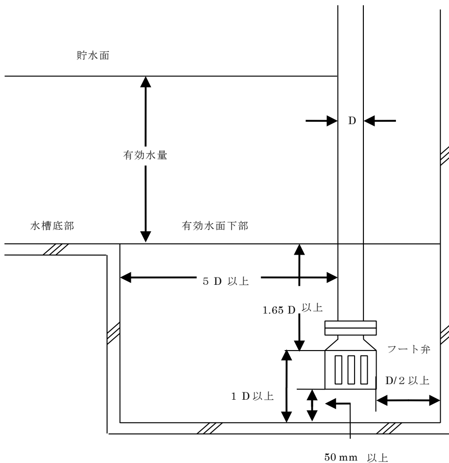
第13-5-1図（地下又は床下水槽を用いサクションピットを設ける場合）
