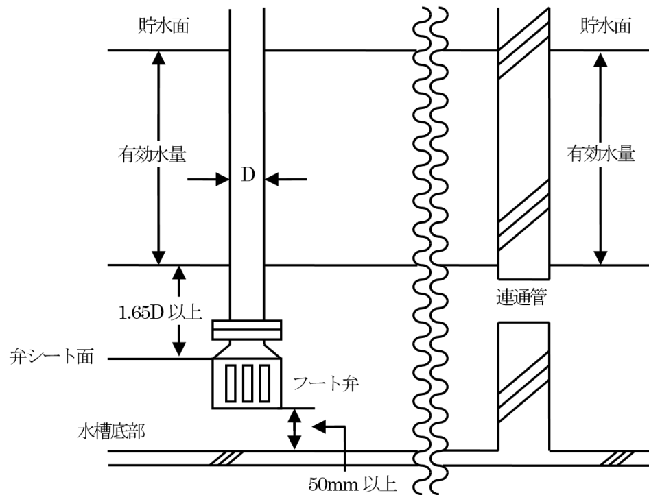
第 1 3 - 5 - 2 図 （地下又は床下水槽を用いサクションピットを設けない場合又は連通管を設ける場合）
