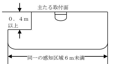
第24-31図 (主たる取付面以外の面の方が高く、かつ、その幅が1.5 m以上である場合)
