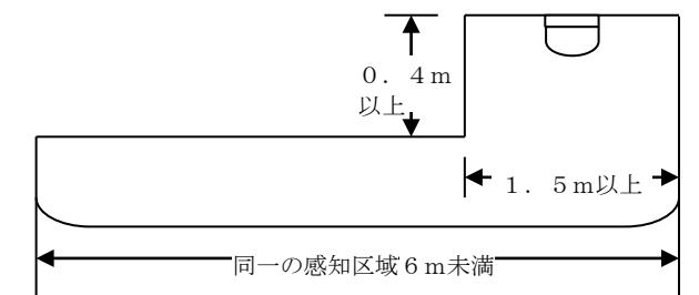
第24-31図 (主たる取付面以外の面の方が高く、かつ、その幅が1.5 m以上である場合)
