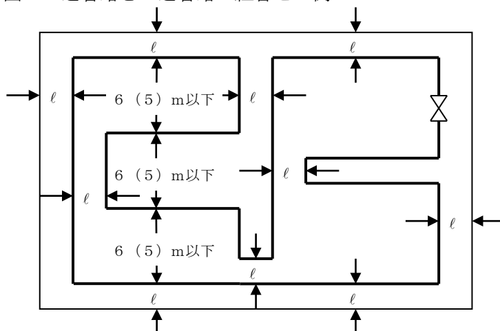
第24-67図 一辺省略と二辺省略の組合せの例1
