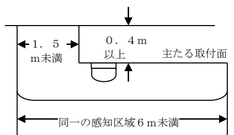
第24-30図 (主たる取付面以外の面の方が高く、かつ、その幅が1.5 m未満である場合)
