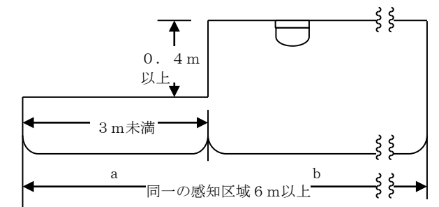
第24-32図 (主たる取付面以外の面の方が低く、かつ、その幅が3 m未満である場合)
