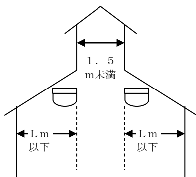
第24-42図 (断面図)
