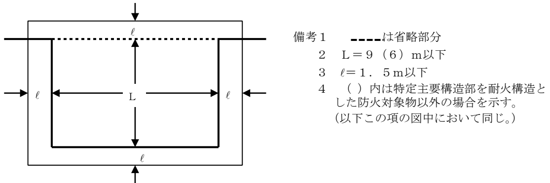
第24-63図 一辺省略の例1
