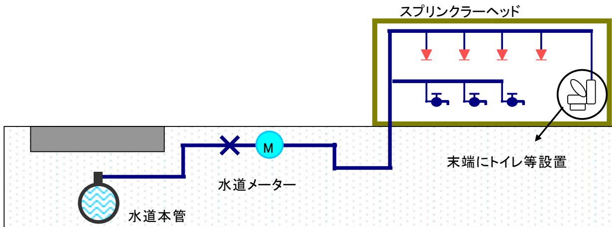
水道直結式スプリンクラー設備設置の配管例
