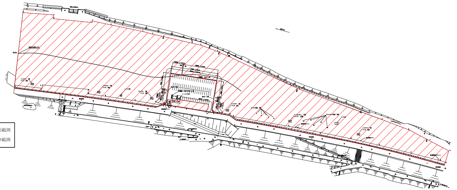
紀の川第9緑地(上流) 平面図 S=1:3000 (A3)
