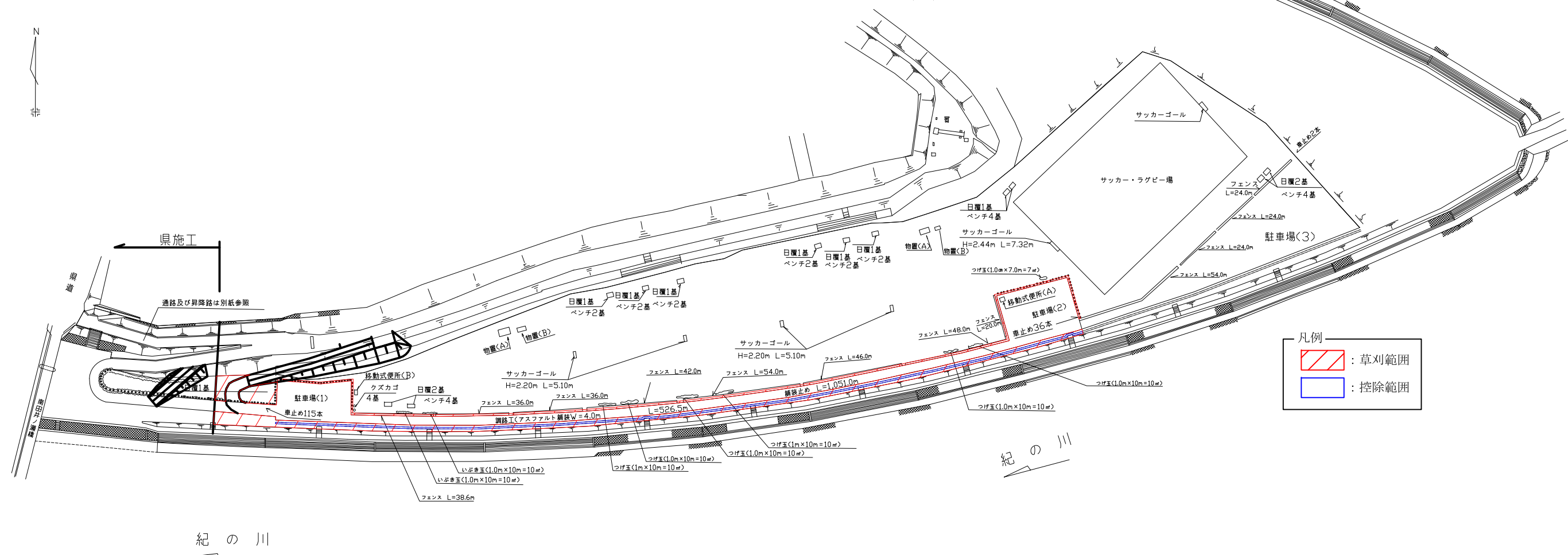
紀の川第7緑地(広場、道路沿い) 平面図 S = 1 : 2000 (A3)
