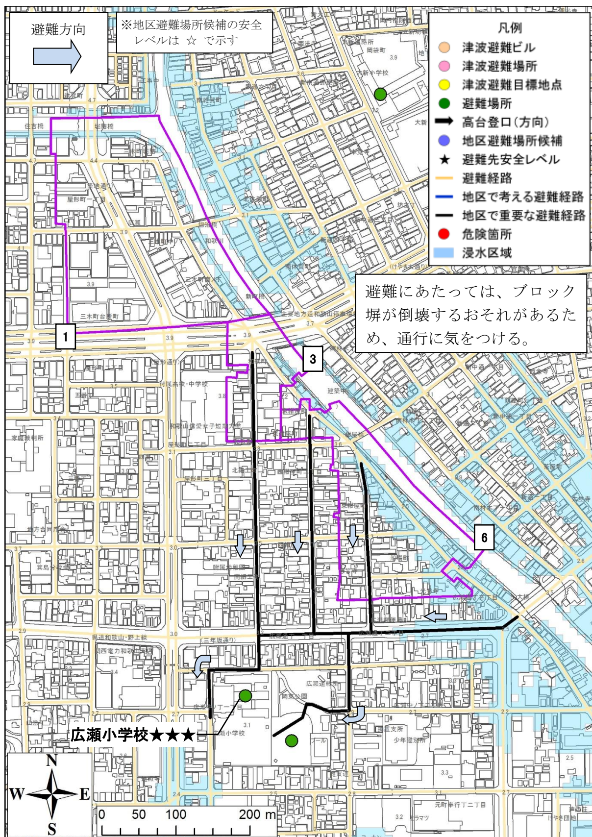
図 8 第1、3、6区検討結果図
