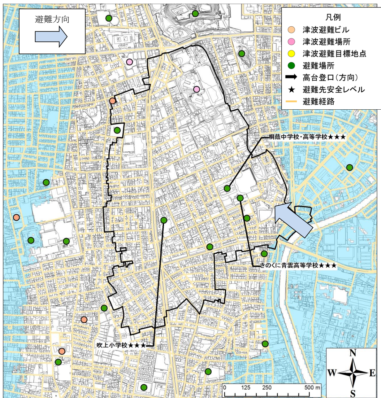
図 4 避難経路図
