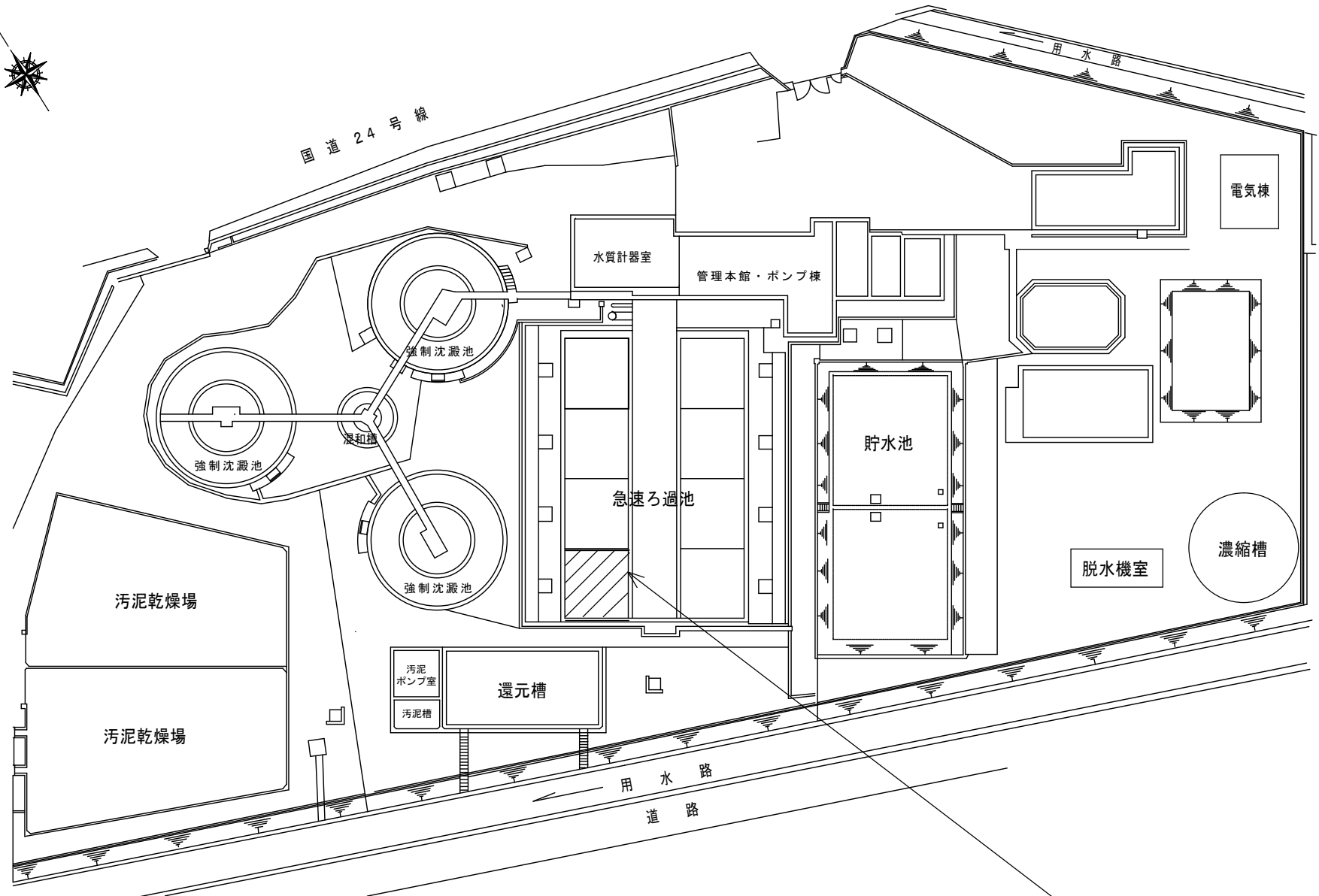
出島浄水場平面図
