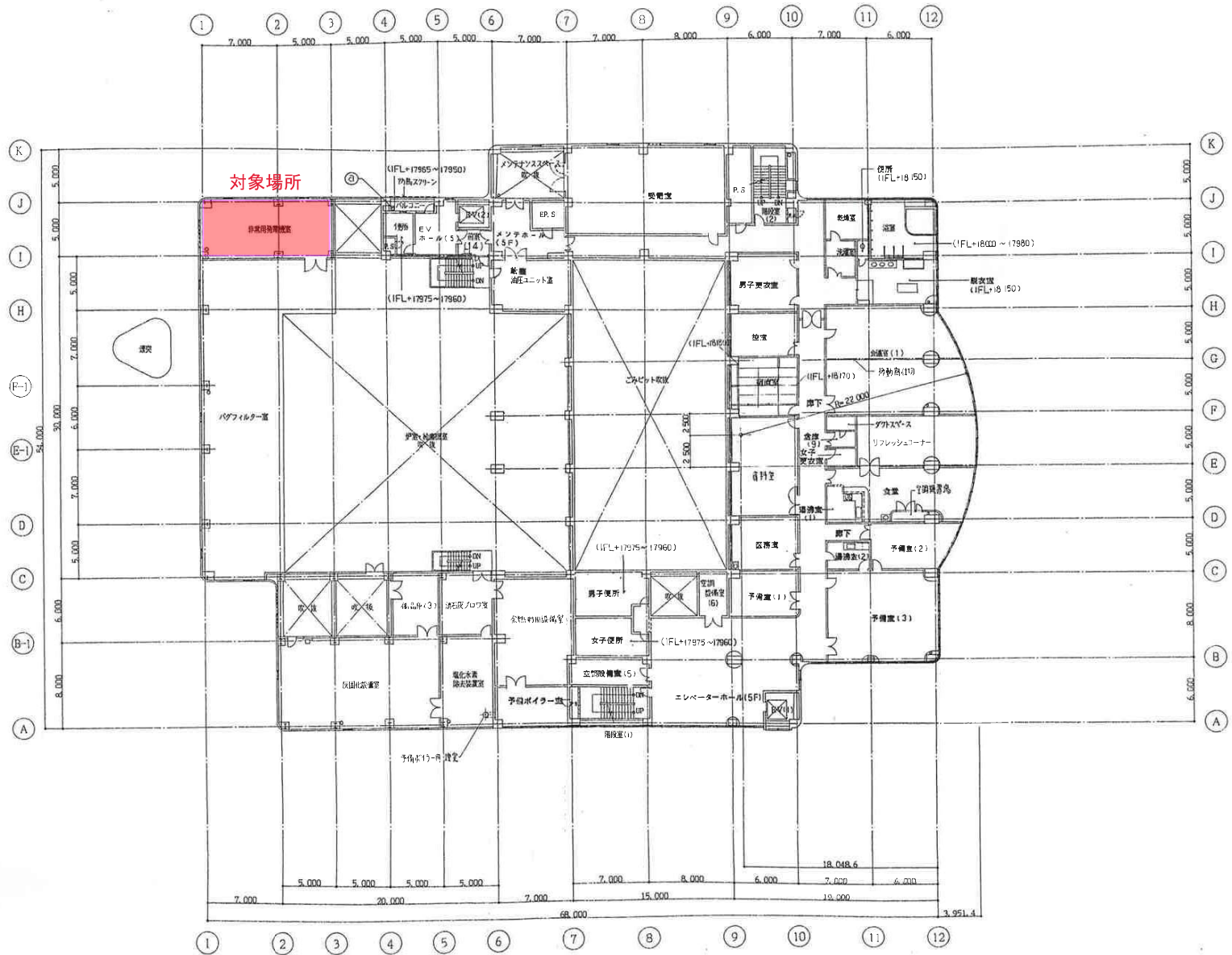
5階 平面図 SFL=IFL+18000
