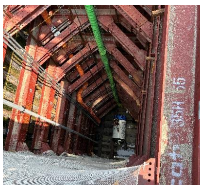
【シールドマシン搬入状況②】
