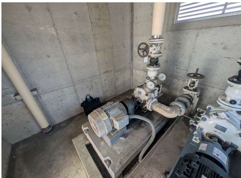
防振継手 (吐出側)
