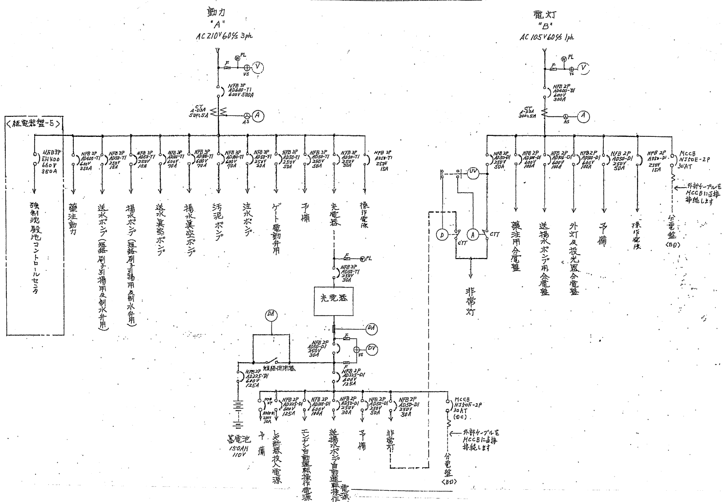
低壓主回路單線接續圖
