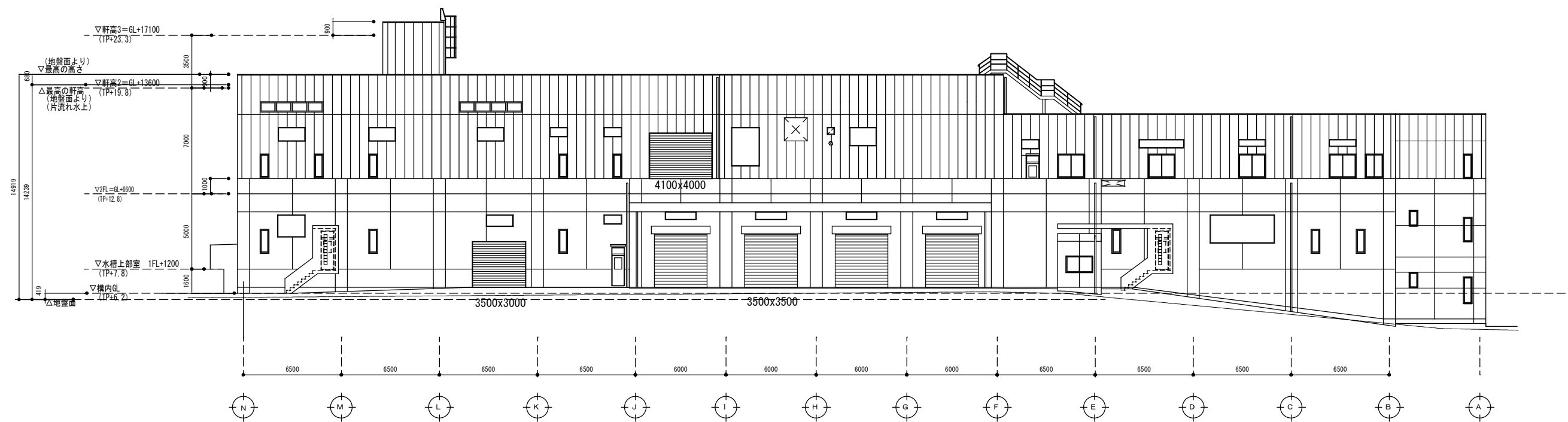
西側 立面図
