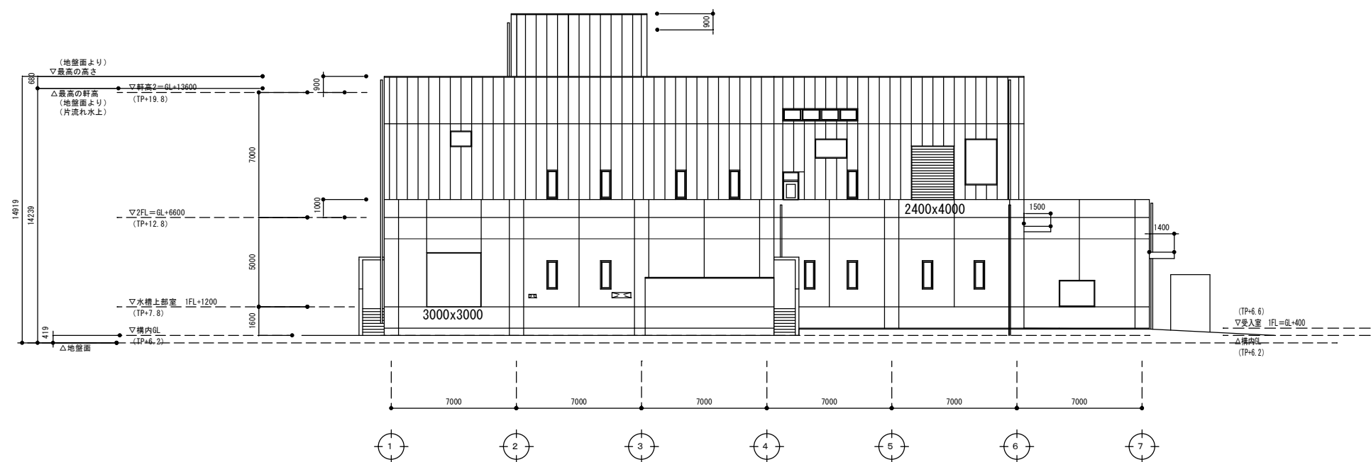
北側 立面図
