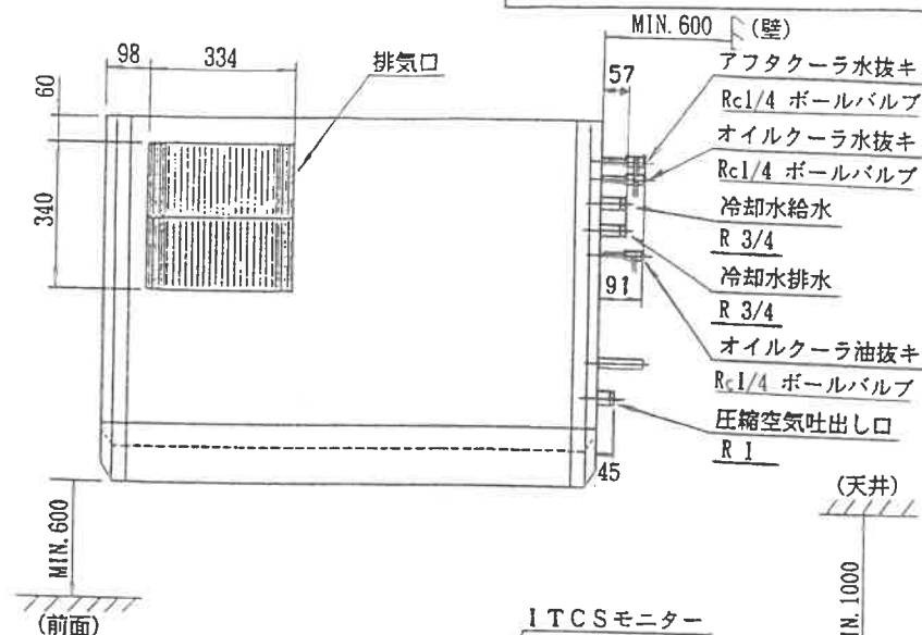
K S T 2 2 W - 6 s M 形 空 気 圧 縮 機 外 形 寸 法 図
